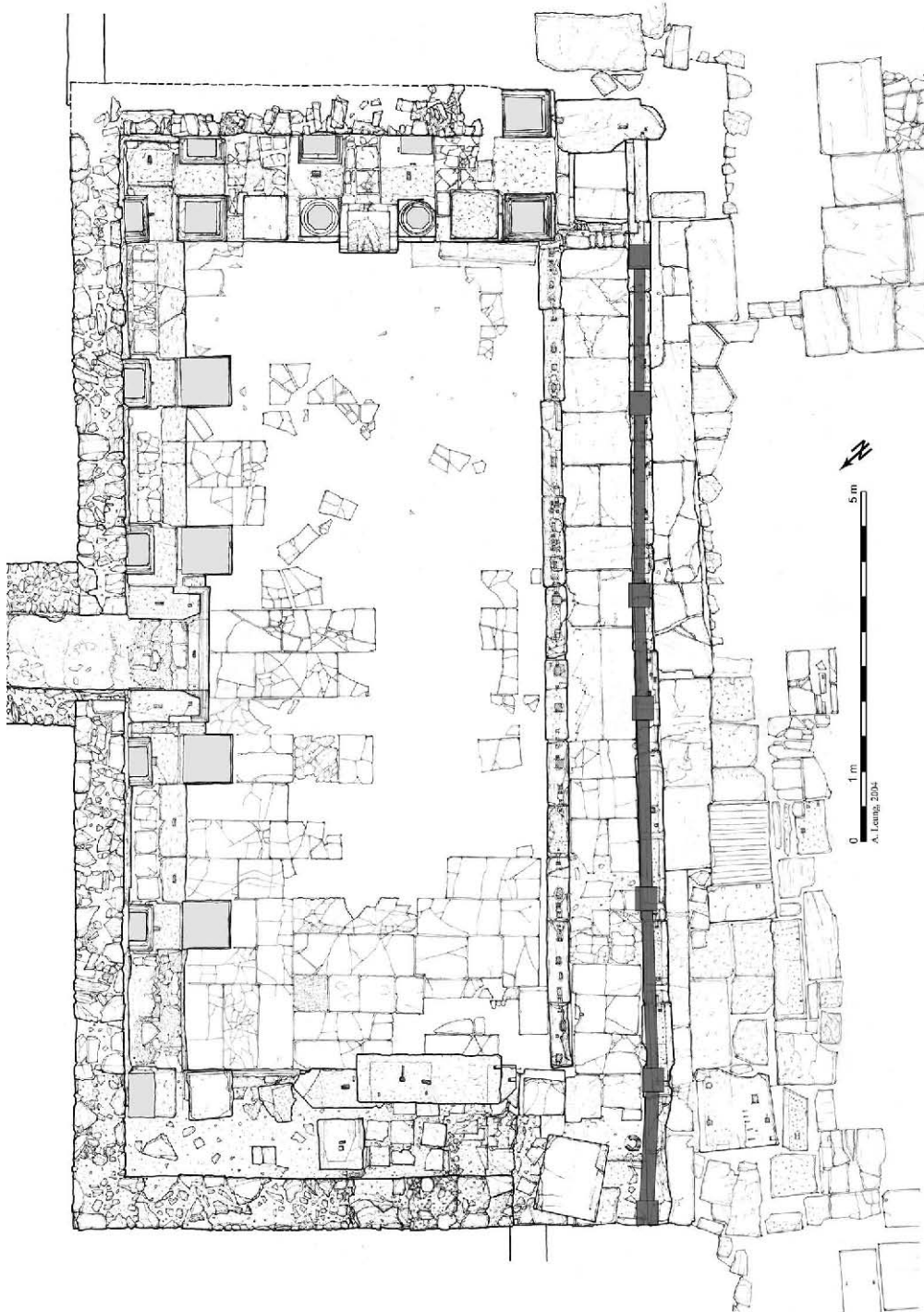
Bestandsplan des Nymphaeum Traiani mit rekonstruierten Positionen der Hermenpfeiler und Schrankenplatten (Zeichnung A. Leung, 2004)
